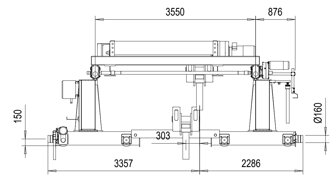
VIEW A-A
